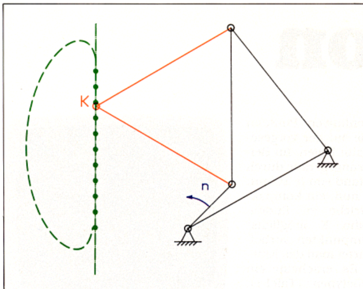
Bild 2: Viergelenkgetriebe das in einem Bereich von mindestens 100 mm eine Gerade fahren soll
