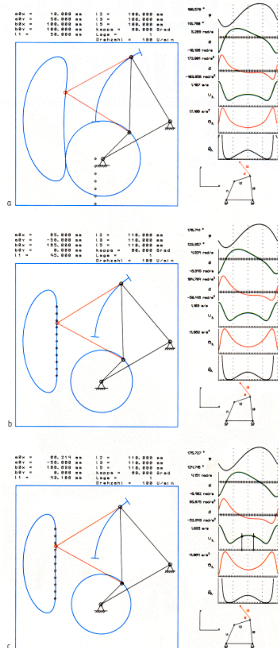
Bild 3: Verschiedene Stufen bei der Computeroptimierung des Getriebes gemäß Bild 2 a Voroptimiertes Getriebe, die flache Bucht der Koppelführung soll zu einer Geradföhrung werden, b in Optimierungsläufen ergab sich die Startvorgabe für eine rechnerische Optimierung, c Endausführung nach rechnerischer Optimierung
